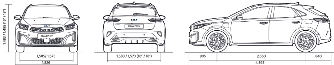
Mitat bensiini/diesel GT-line ja PHEV (mm)
